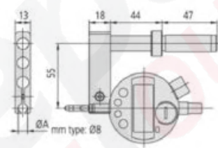
12AAA792 (avec comparateur en option)
